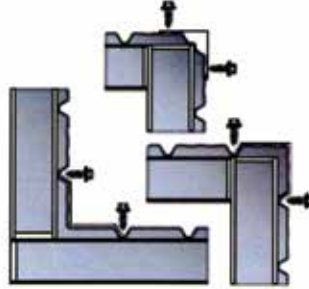
BUITEN- EN BINNENHOEKEN
