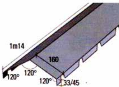
GETANDE NOKKEN
