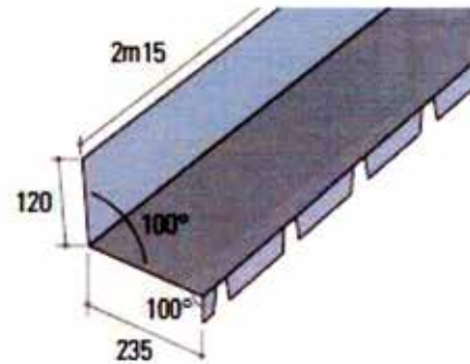
OPSTAANDE GETANDE MUURNOKKEN
