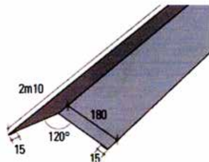
PLATTE NOKKEN
