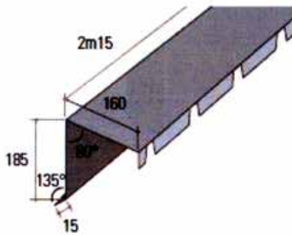
GETANDE MUURNOKKEN
