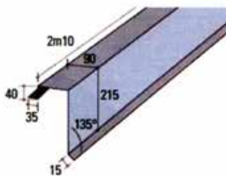
WINDVEREN
